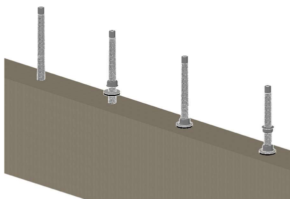
Rys. schemat kolejnych etapów montażu śruby dwugwintowej
