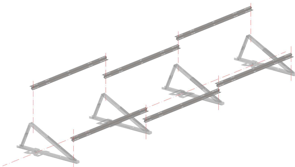
Rys. Schemat poglądowy rozmieszczenia płatwi
