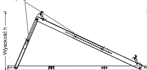
Ramię regulowane
