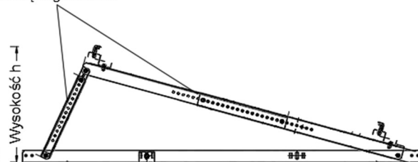
Ramię regulowane
