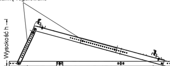
Ramię regulowane
