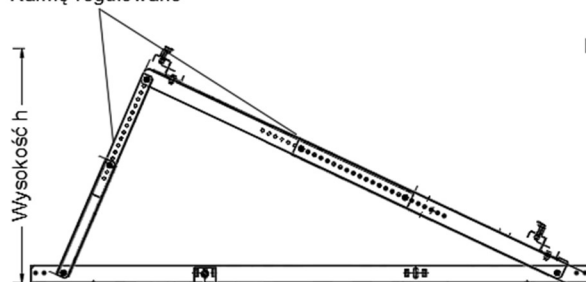
Ramię regulowane
