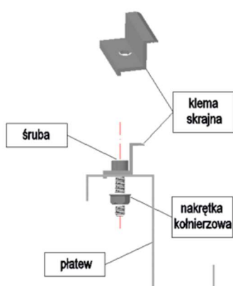
Rys. Schemat poglądowy wstępnego montażu klem
